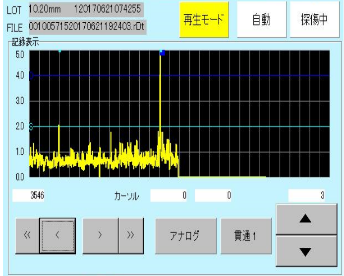
探傷不良品波形圖
