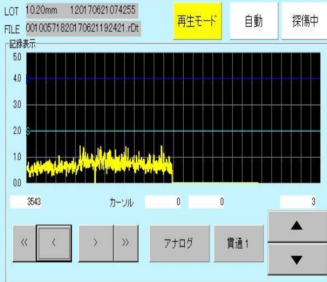
探傷良品波形圖
