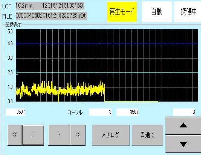
探傷良品波形圖
