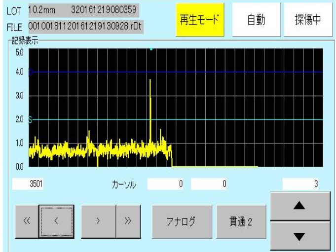
探傷不良品波形圖
