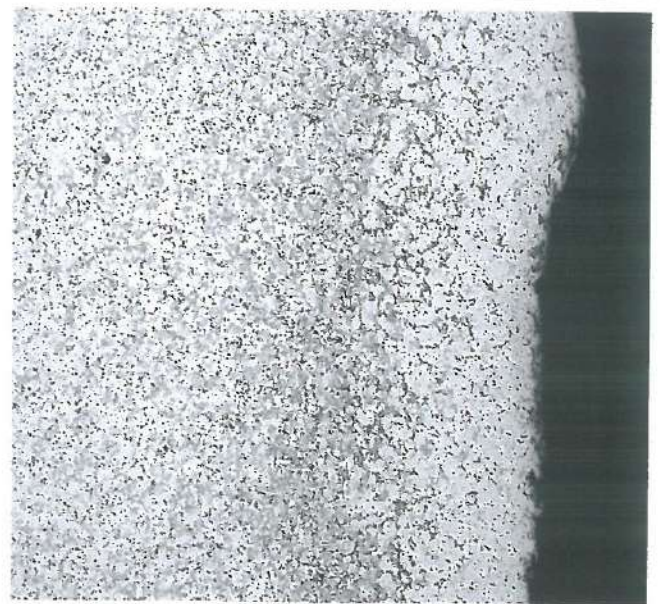
圖(6)表面不良樣品金相橫切面 200X Picral
