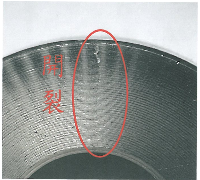
圖(2) 開裂樣品外觀_X10
