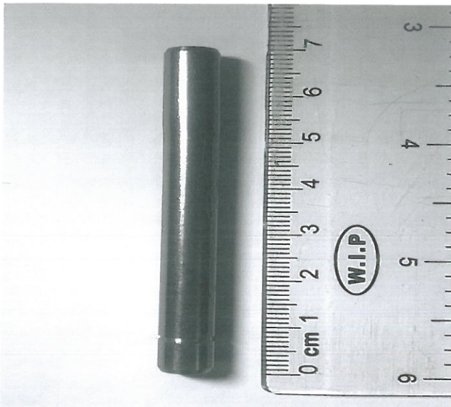
圖(1) 開裂樣品外觀
