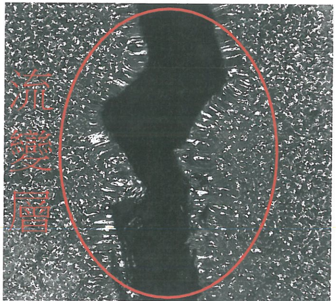
圖(4) 開裂樣品金相橫切面 200X Picral
